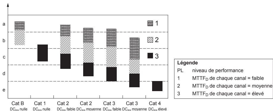
Figure 5 - Relation entre les catégories, le DC avg , le MTTFD de chaque canal et le PL.
